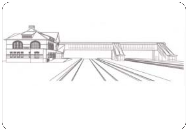
Den optimala lösningen på spårläggningen vid Alvesta station skulle kunna se ut som den Leif Johansson skissat. Maximal säkerhet vid förbipassage genom grupper om tre spår. Mittspåret används för genomgående trafik och för förbigång av stillastående tågsätt. En lösning som hör framtiden till och kunde bli en framtida förebild.
